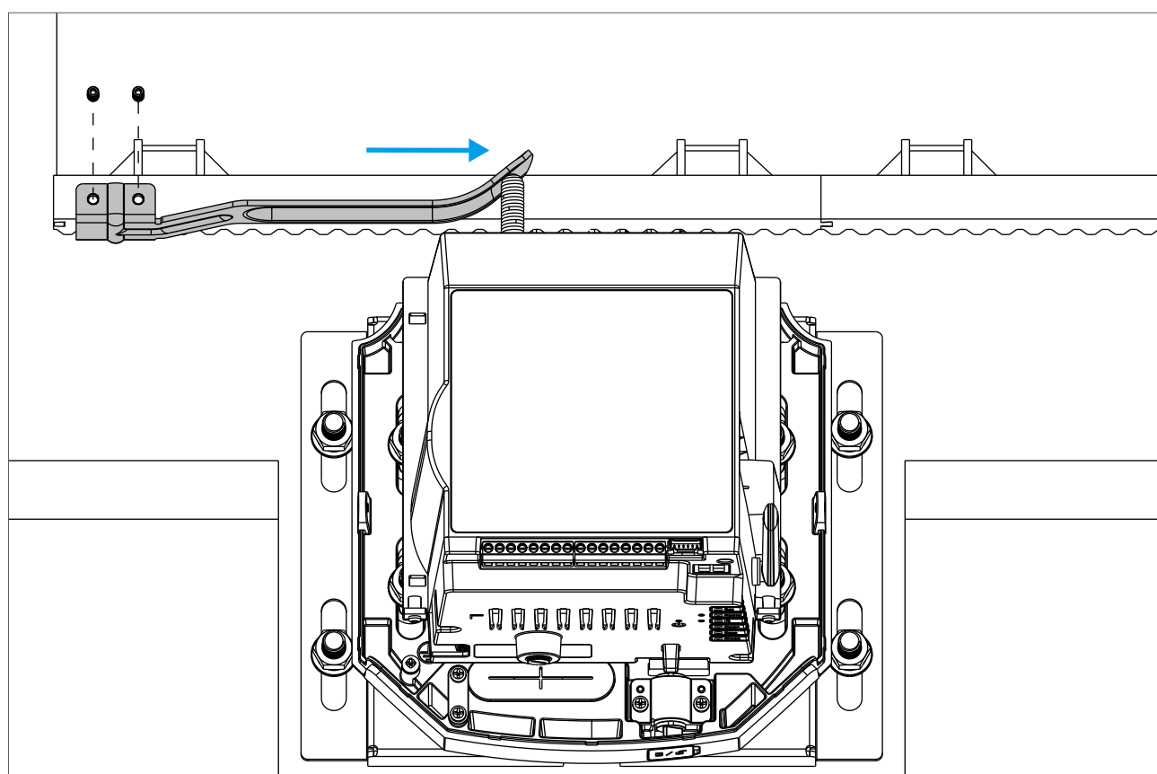
Popravite lim leve granice
